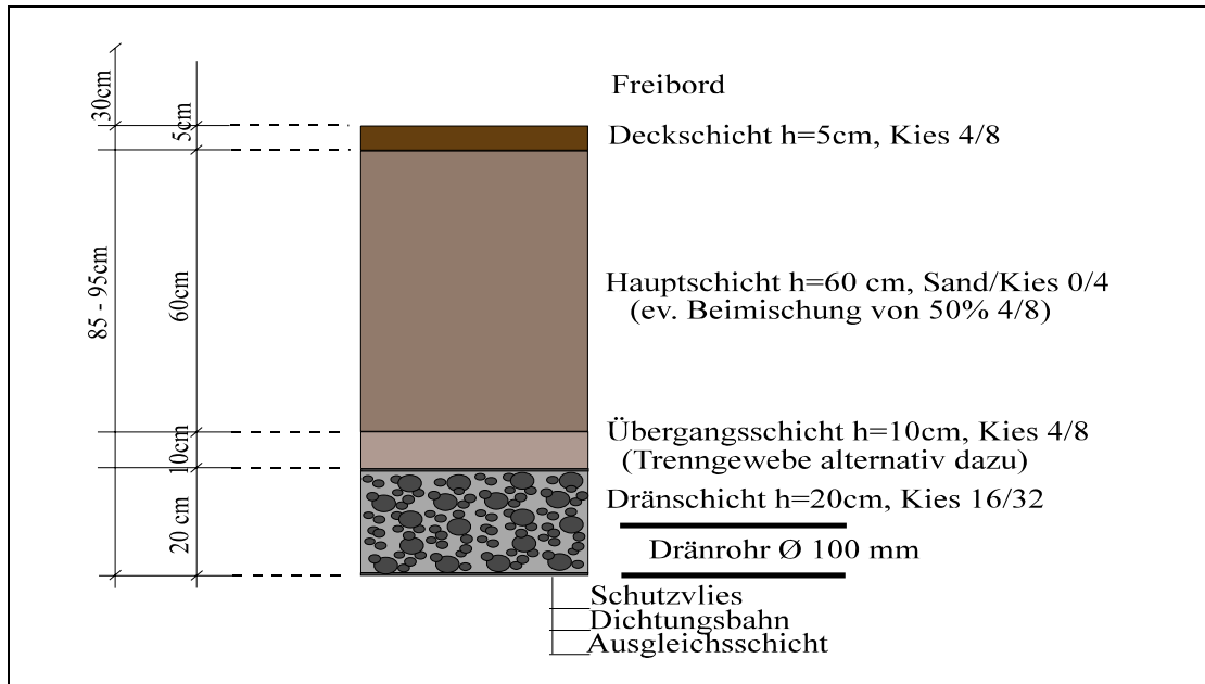
Abb. 7.2-3: Bodenprofil eines vertikal durchströmten bepflanzten Bodenfilter nach ÖNORM B 2505 (2003)
