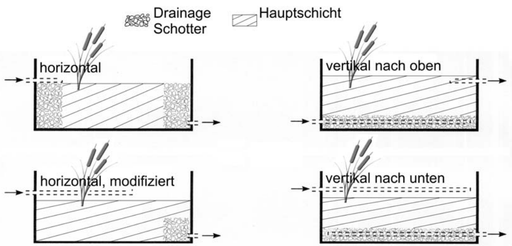
Abb. 7.2-1: Hydraulische Durchströmung unterschiedlicher Bauformen
