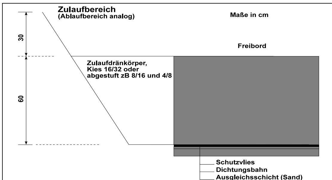
Abb. 7.2-4: Bodenprofil eines horizontal durchströmten bepflanzten Bodenfilter nach ÖNORM B 2505 (2003)
